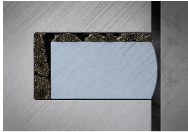
Şek. 1: Segman yuvasında kir birikmesi
