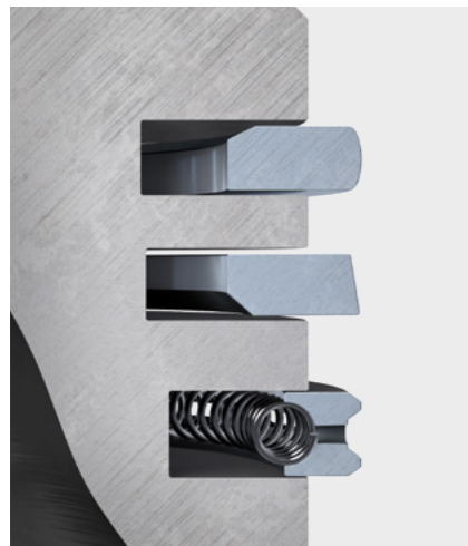
Şek. 2: Gerilmemiş durumdaki piston segmanları – Torsiyon henüz etkili değil
