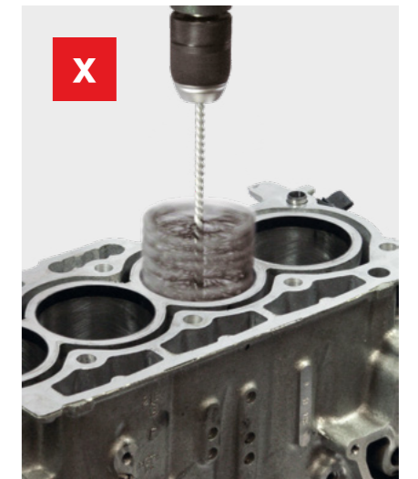
Şek. 3: Honlama fırçaları
