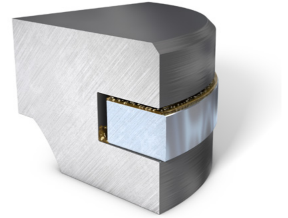
Şek. 2: Segman yuvasındaki kirler ve yağ tortuları birikerek aşındırıcı bir macun haline gelir.
