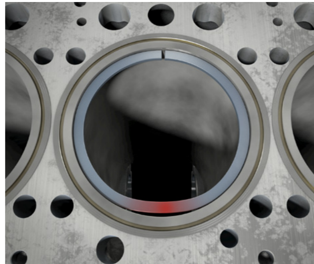
Şek. 2: Aşırı çekme nedeniyle orak şeklinde yarıklar (boşluklar) oluşması
