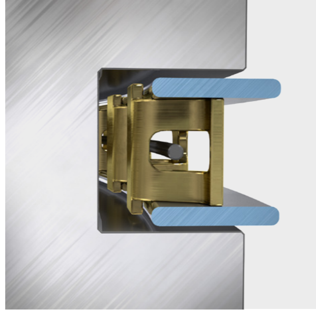
Üç parçalı yağ sıyırma segmanı
