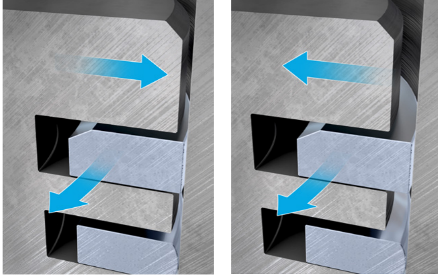
Piston segmanının radyal hareketi
