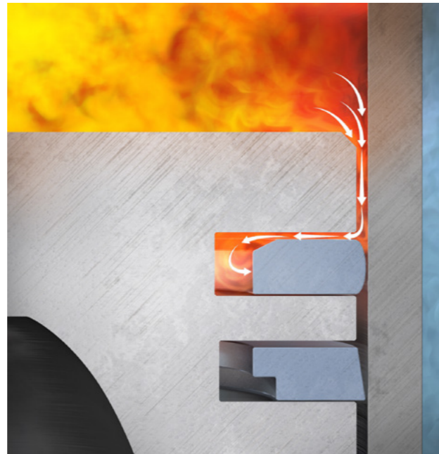
Yanma gazları sızdırmazlığının sağlanması
