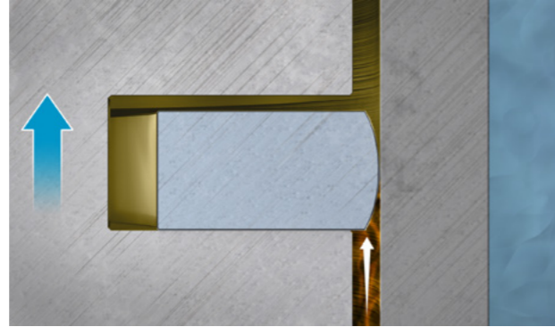
Şek. 1: Yuva kanadı ile sızdırmazlık
