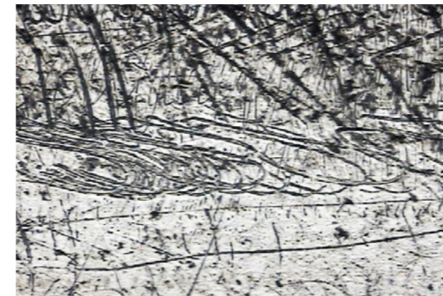
Şek. 4 ve 5: Üst segman kenarındaki yuvarlanma izlerine örnekler
