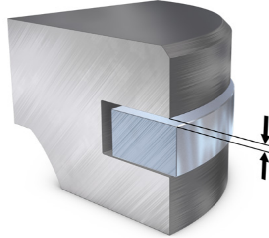
Şek. 1: Segman yükseklik boşluğu
