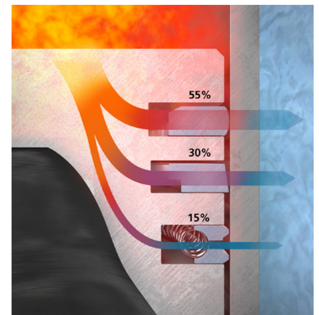
Isı iletimi
