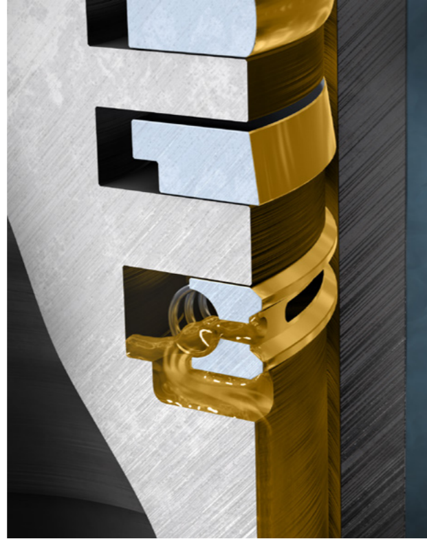
Yağ sıyırma segmanı
