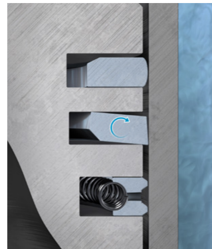
Şek. 4: Negatif torsiyon
