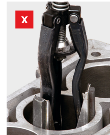
Şek. 2: Yaylı honlama taşları
