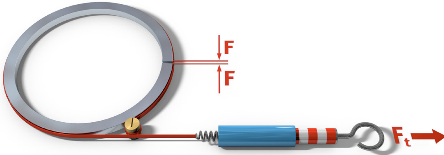
Şek. 1: Teğetsel kuvvet ölçümü
