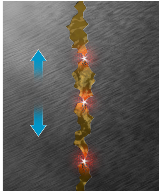
Şek. 1: Karışık sürtünme – Piston segmanı ve silindir duvarı arasında metalik temas
