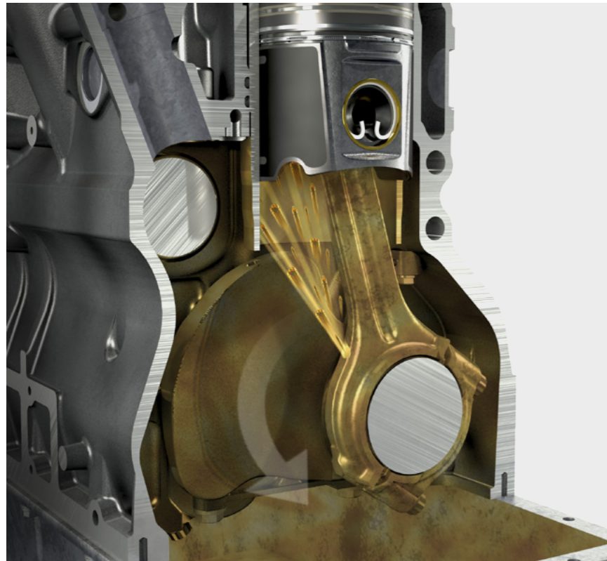
Şek. 1: Biyeldeki yağ sıçratma delikleri, çalışma yüzeyinin yağlanmasını garanti eder
