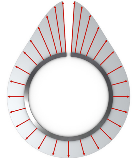
Şek. 3: Pozitif-oval radyal basınç dağılımı
