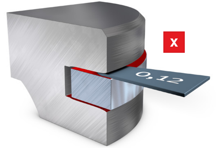
Şek. 2: Aşınmış segman yuvası
