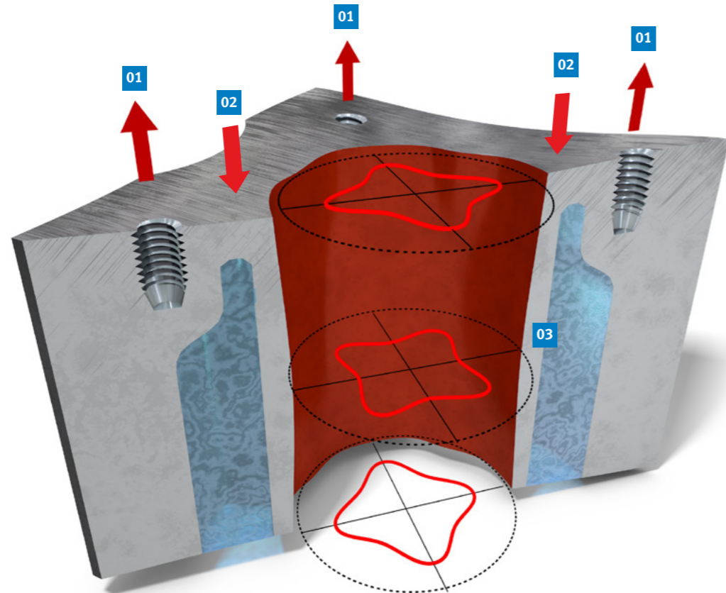
Şek. 1: 4. derece silindir çekmesi
