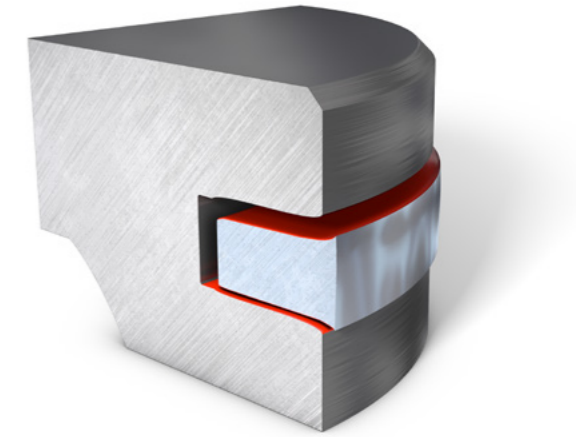
Şek. 3: Aşınma sonucu yüksekliği azalan piston segmanı nedeniyle piston segmanı oluğu genişler
